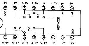
各集成块引脚电压
